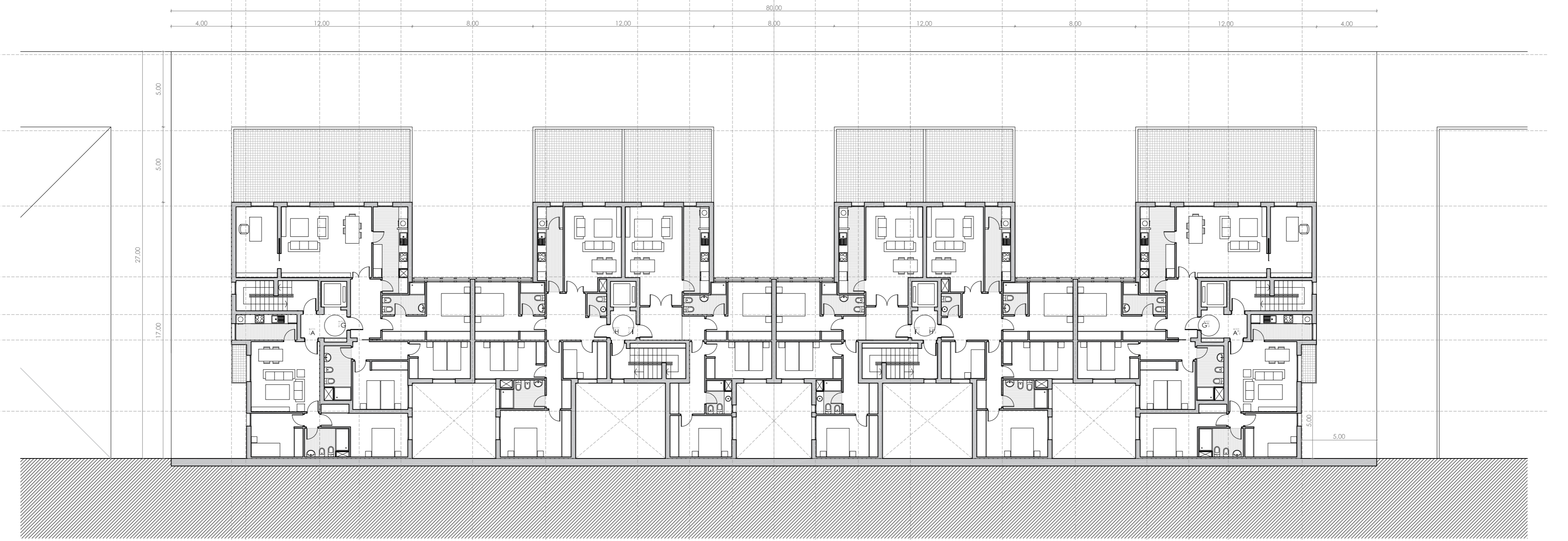
NIVEL 5 cota +17.40
