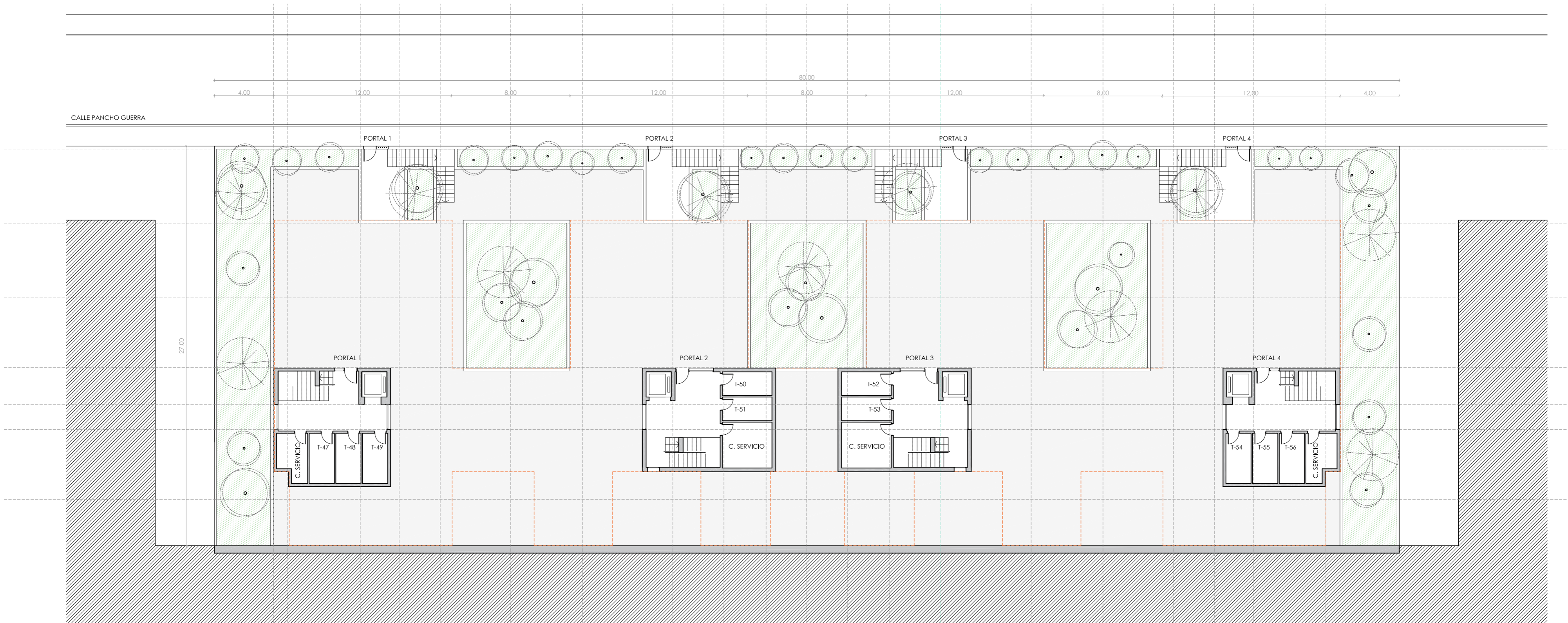
NIVEL 1 cota +4.00
