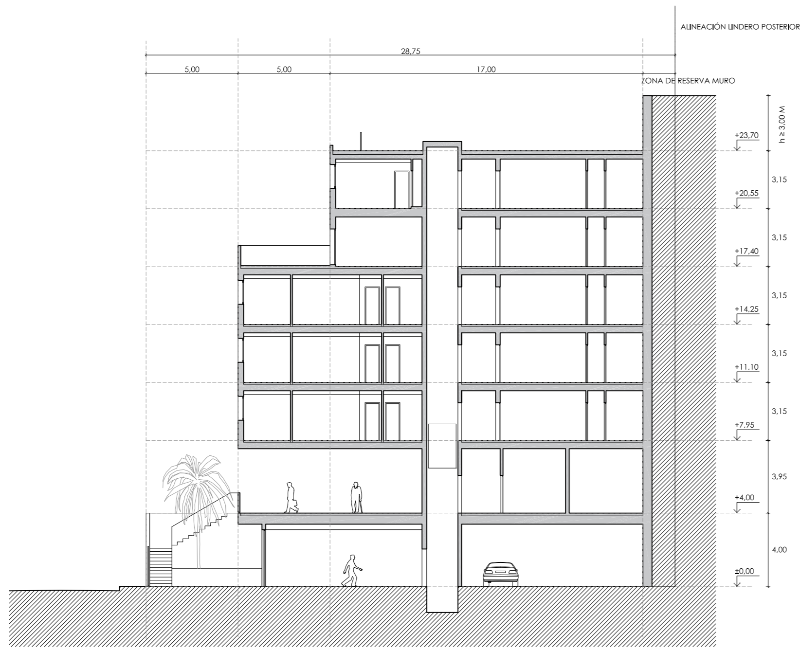
SECCIÓN A-A'
