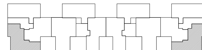
PLANTA NIVEL 6
