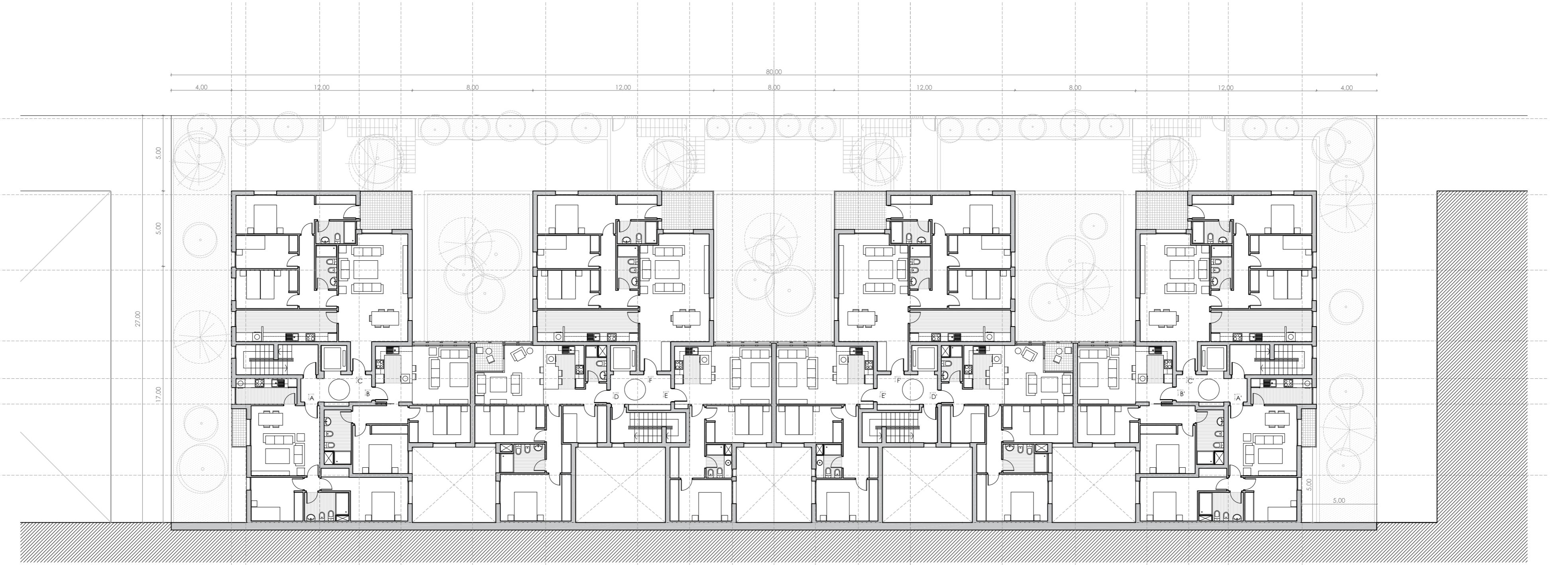
NIVELES 2-3-4 cota + 7.95 cota +11.10 cota +14.25
